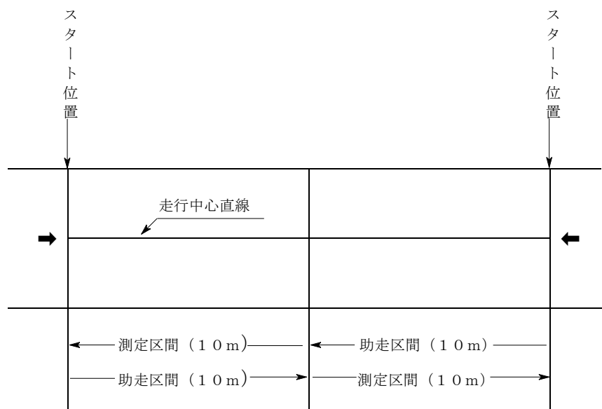
図 最高速度試験
