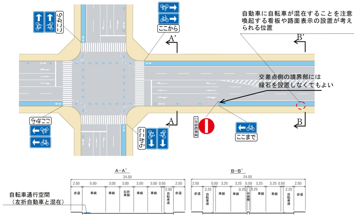
図Ⅱ-54 左折自動車のみ混在の場合の自転車道（自転車一方通行）が交差する交差点の例
