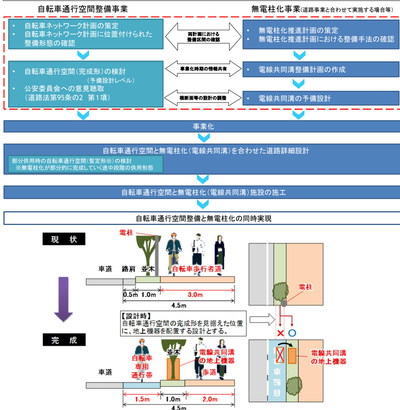
図 I-15 無電柱化（電線共同溝）事業との連携イメージ
