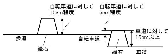
図Ⅱ-10 自転車道の断面構造の例
