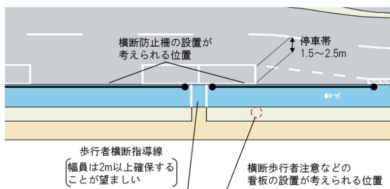
図Ⅱ-39 自転車道のある道路に停車帯を設置する例
