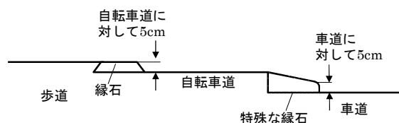
図Ⅱ-10 自転車道の断面構造の例
