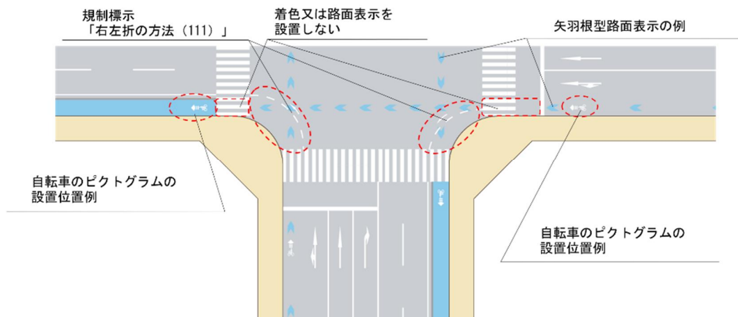
図Ⅱ-55 左折自動車のみ混在の場合の交差点隅角部の道路構造の例（自転車道（自転車一方通行）の場合）
