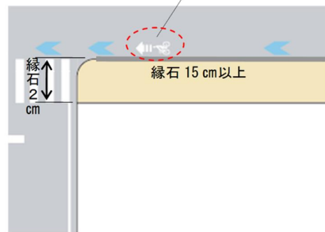
図Ⅱ-76 交差点隅角部の道路構造の例（車道混在の場合）
