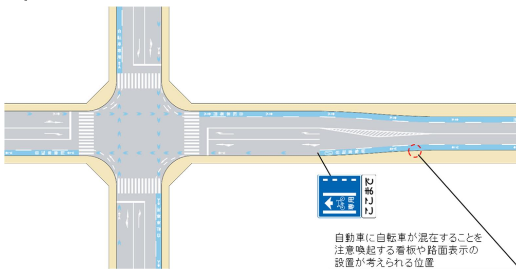
図Ⅱ-46 左折自動車のみ混在の場合の車道混在を注意喚起する看板・路面表示の位置の例（自転車専用通行帯の場合）
