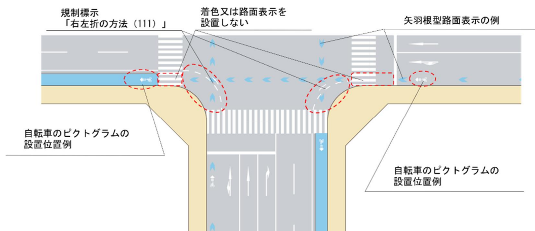
図Ⅱ-62 左折自動車のみ混在の場合の交差点隅角部の道路構造の例
