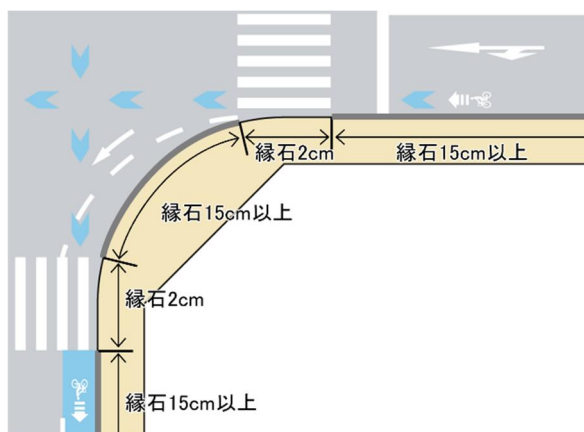
図Ⅱ-47 左折自動車のみ混在の場合の交差点隅角部の縁石構造の例（自転車専用通行帯の場合）
