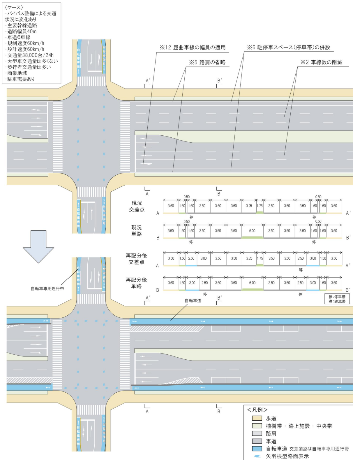
図Ⅱ-13 幅員 40m の道路において空間の再配分により自転車道を確保する例
