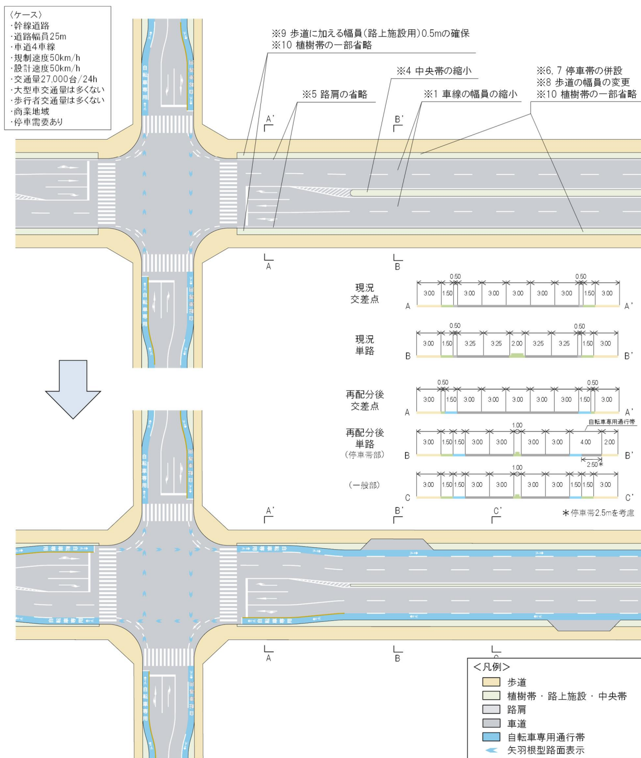
図Ⅱ-19 幅員 25m の道路において空間の再配分により自転車専用通行帯を確保する例
