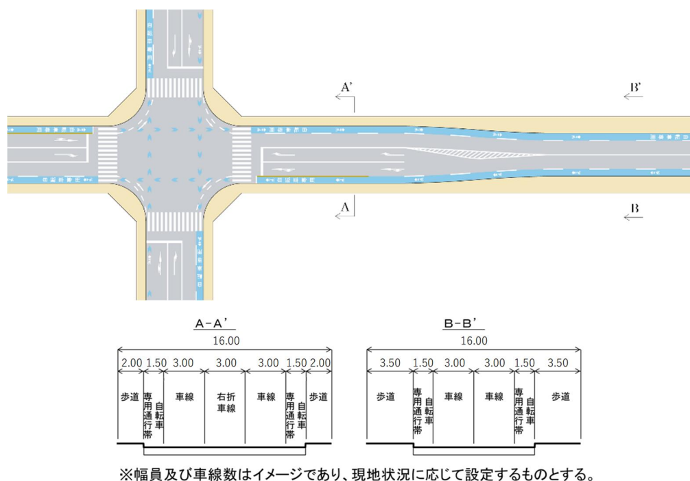
図Ⅱ-63 分離の場合の自転車専用通行帯が交差する交差点の例
