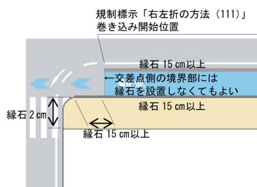
図Ⅱ-70 交差点隅角部の道路構造の例
