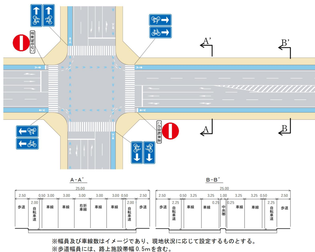
図Ⅱ-58 分離の場合の自転車道（自転車一方通行）が交差する交差点の例
