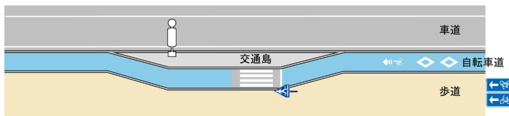
図Ⅱ-26 車道と自転車道との間に交通島のバス停留所を設ける例（島型） （バス交通が多く道路空間に余裕がある路線）
