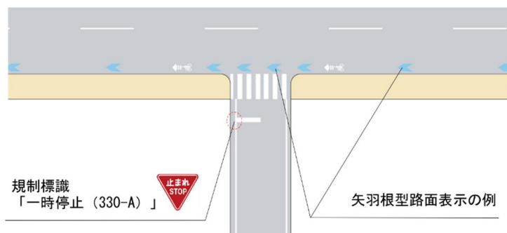
図Ⅱ-75 交差点イメージ（車道混在の場合）
