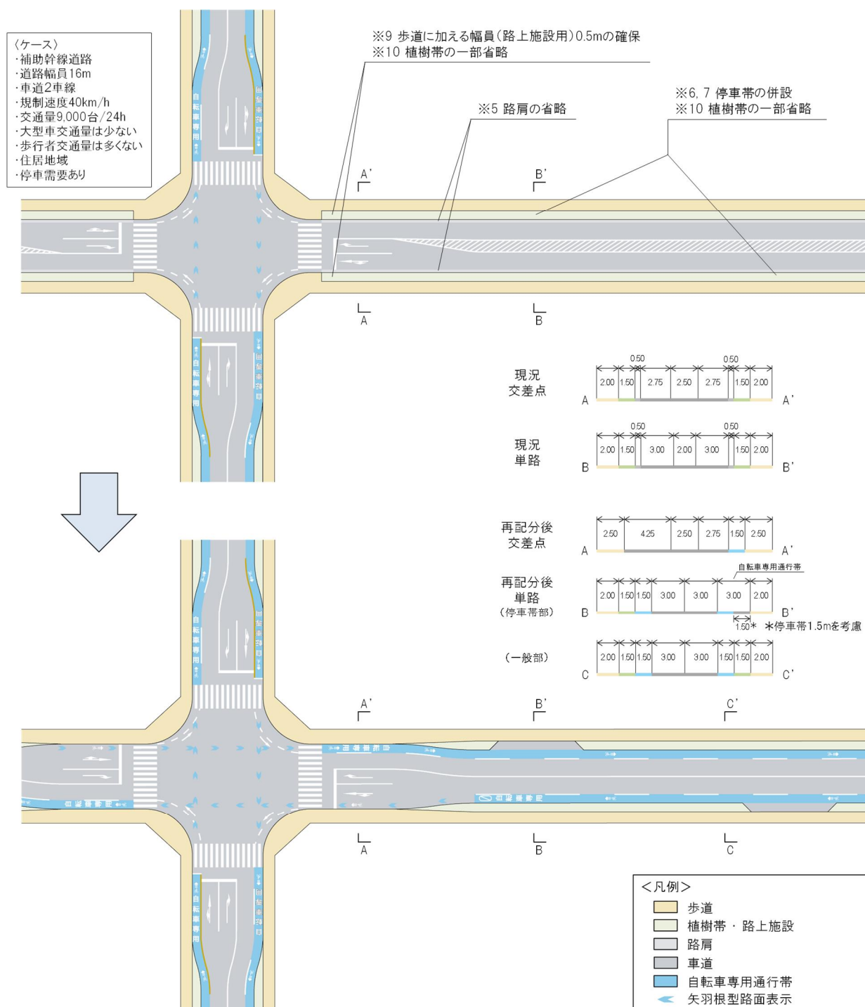
図Ⅱ-16 幅員 16m の道路において空間の再配分により自転車専用通行帯を確保する例
