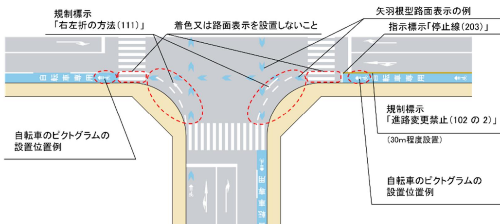
図Ⅱ-64 分離の場合の交差点隅角部の道路構造の例 (自転車専用通行帯の場合)
