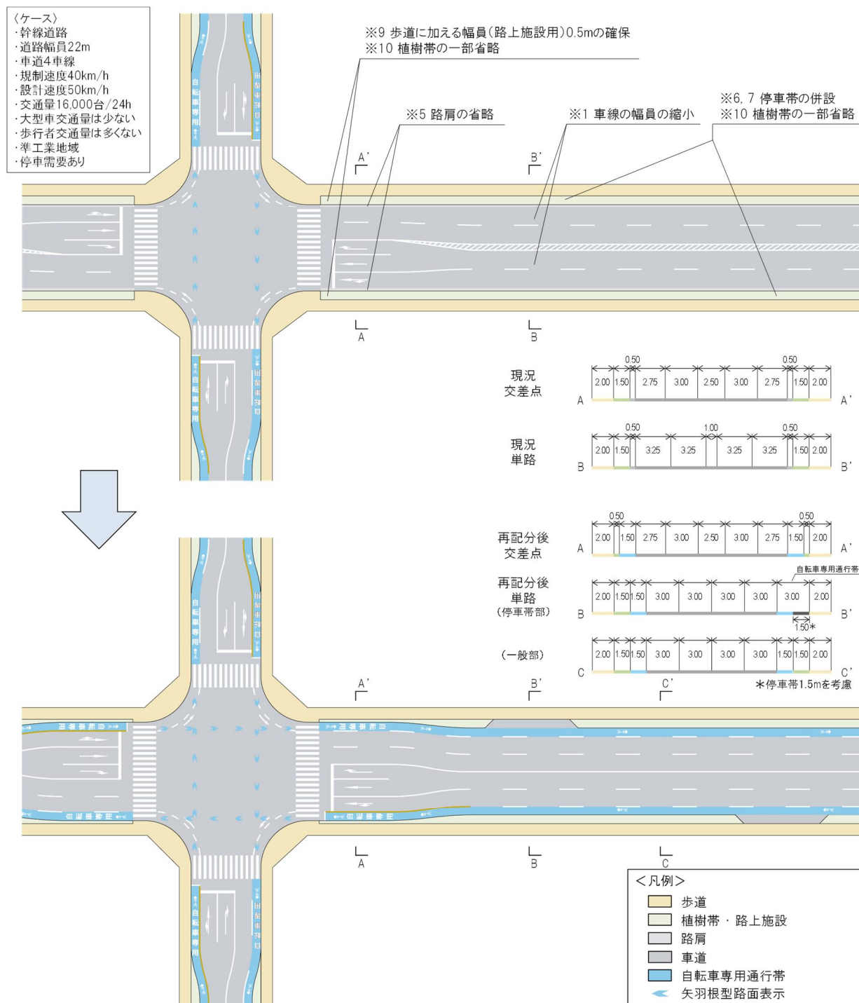
図Ⅱ-18 幅員 22m の道路において空間の再配分により自転車専用通行帯を確保する例
