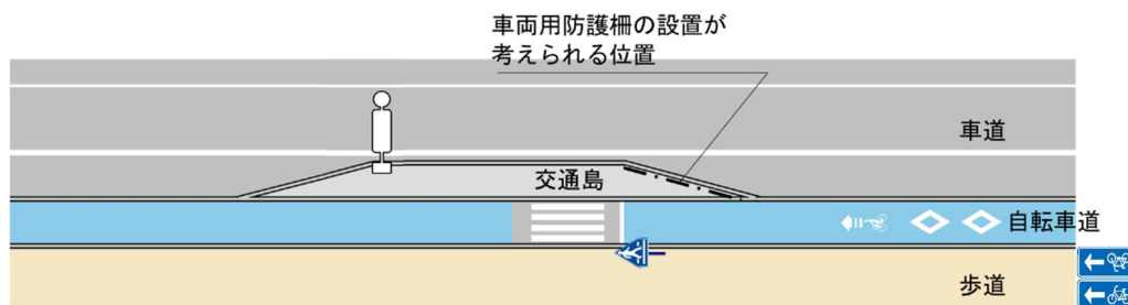
図Ⅱ-27 車道と自転車道との間に交通島のバス停留所を設ける例（テラス型） （バス交通が多く道路空間に余裕がある路線）
