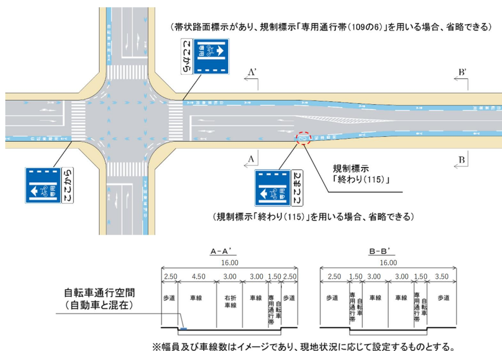
図Ⅱ-61 左折自動車のみ混在の場合の自転車専用通行帯が交差する交差点の例
