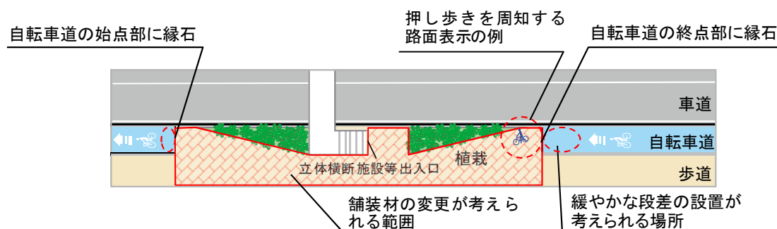
図Ⅱ-36 立体横断施設等出入口付近で自転車道を歩道に接続する例
