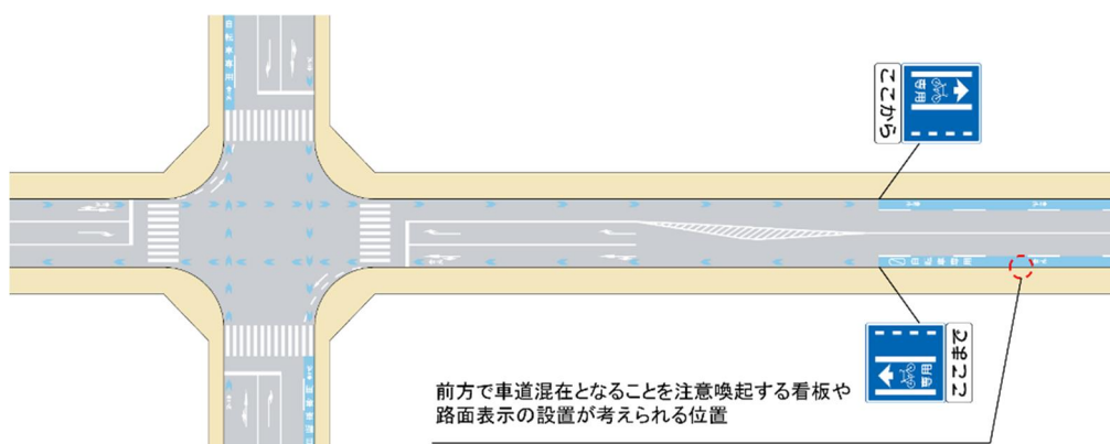
図Ⅱ-53 混在の場合の車道混在を注意喚起する看板・路面表示の位置の例 (交差点流出側に自転車専用通行帯を確保できない場合)
