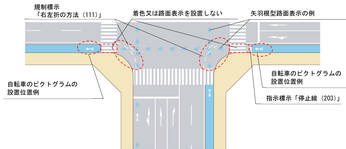
図Ⅱ-59 分離の場合の交差点隅角部の道路構造の例 (自転車道（自転車一方通行）の場合)
