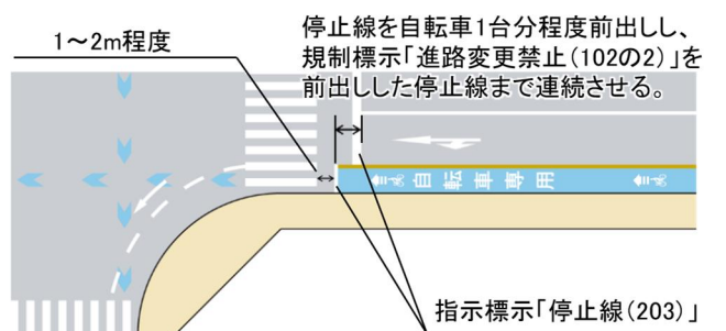
図Ⅱ-49 停止線の前出しの例 (自転車専用通行帯の場合)
