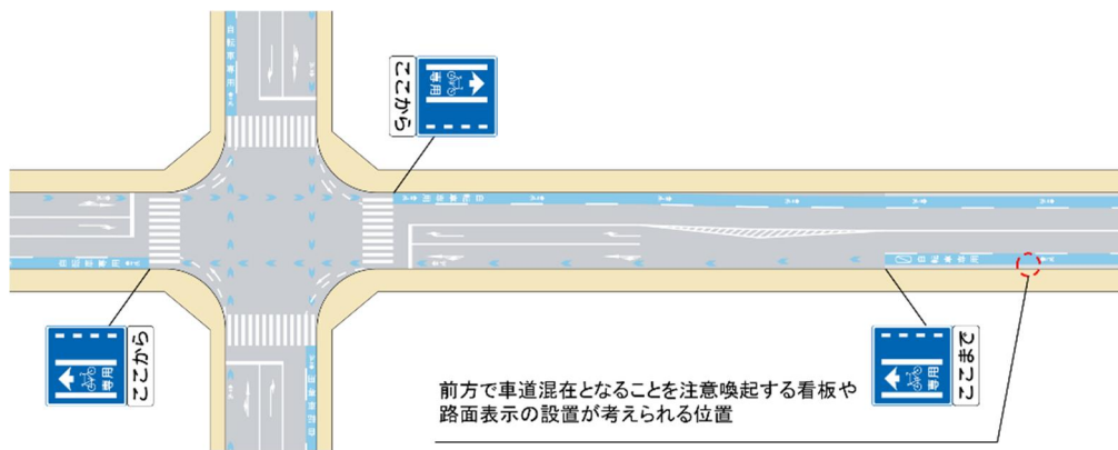
図Ⅱ-52 混在の場合の車道混在を注意喚起する看板・路面表示の位置の例 (交差点流出側に自転車専用通行帯を確保可能な場合)
