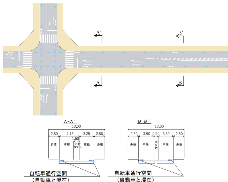
図Ⅱ-67 車道混在が交差する交差点の例
