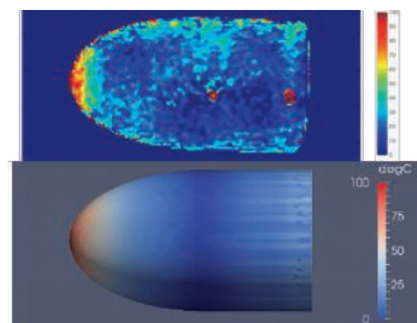
実験計測による温度分布 (上) 数値計算による温度分布 (下)
