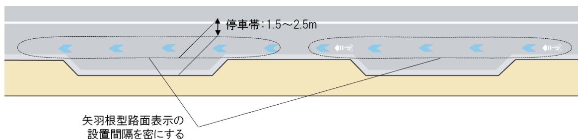
図Ⅱ-42 車道混在の道路に停車帯を設置する例
