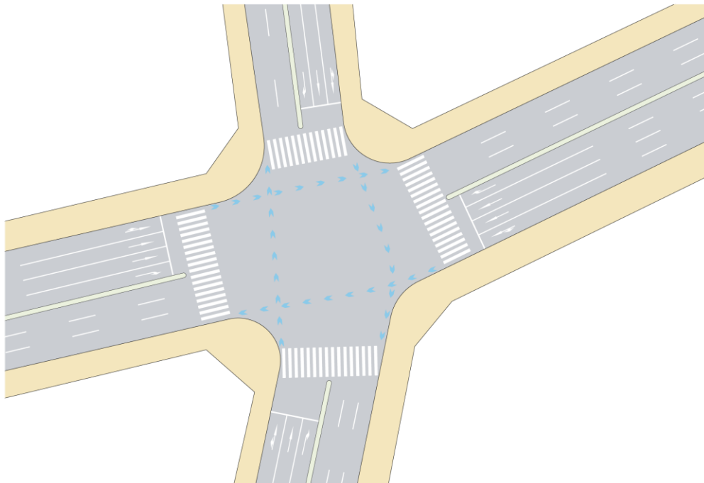
図Ⅱ-81 折れ脚交差点における矢羽根型路面表示の設置例
