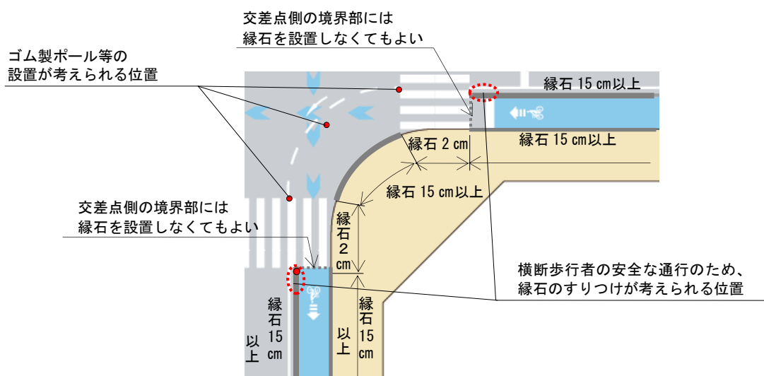
図Ⅱ-59 分離の場合の交差点隅角部の縁石構造の例 (自転車道(自転車一方通行)の場合)
