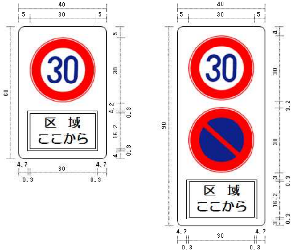
図例(3) 参考規格
