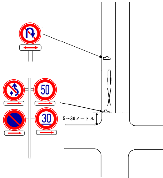
図例(3) 道路標識に代えて道路標示を設置する場合
