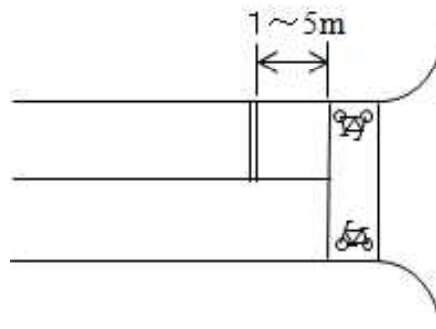
図例(2) 自転車横断帯を単独で設置する場合の停止線の位置
