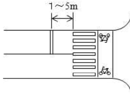
図例(2) 自転車横断帯を単独で設置する場合の停止線の位置
