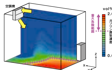
室内に散布されたガソリンの蒸気濃度の計算予測例
