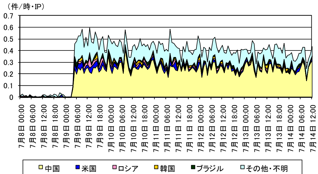
図1 5060/UDP に対するアクセス状況
